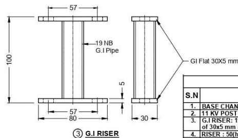
③ G.I RISER
